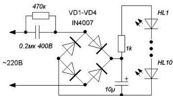
Рисунок 74 – Схема електрична принципова драйвера
