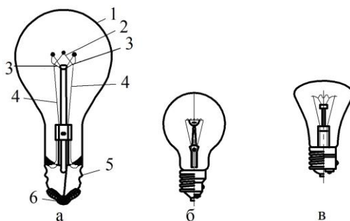
Рисунок 26 - Конструкція ЛР загального призначення:
