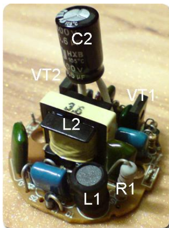
Рисунок 47 – Будова електронного блоку компактної люмінесцентної лампи
