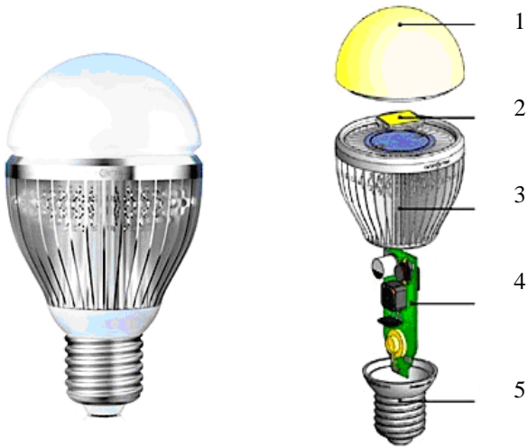
Рисунок 73 - Світлодіодна лампа типу EKF: а) загальний вигляд; б) загальна будова – 1 – розсіювач, 2 – плата із світло діодами (кластер), радіатор, 4 – драйвер, 5 – цоколь
