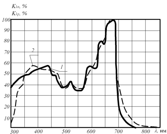
Рисунок 5 – Спектральна чутливість: 1 – середнього листа рослин; 2 – фітометра
