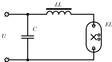
Рисунок 54 – Принципова схема включення чотириелектродних ламп типу ДРЛ: LL – дросель; C – конденсатор; EL – лампа
