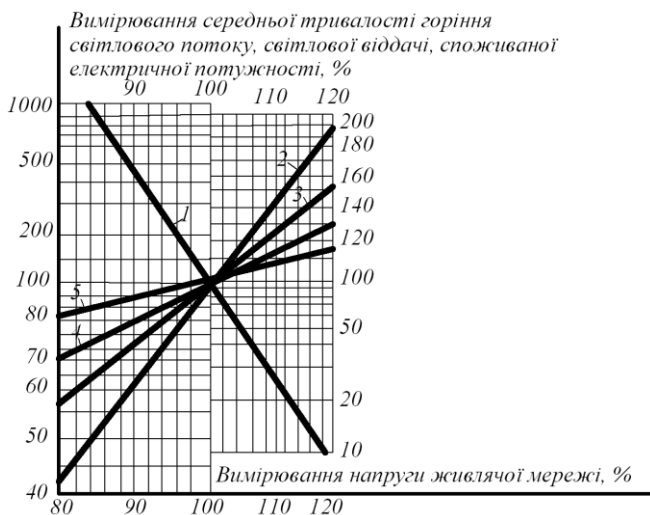
Рисунок 27 – Залежність світлотехнічних, електричних і експлуатаційних параметрів ламп розжарювання загального призначення від зміни напруги живлячої мережі:
