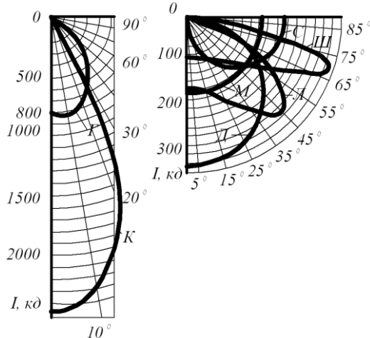
Рисунок 77 - Типові криві сили світла в абсолютних одиницях при світловому потоку джерела світла, який дорівнює 1000 лм:
