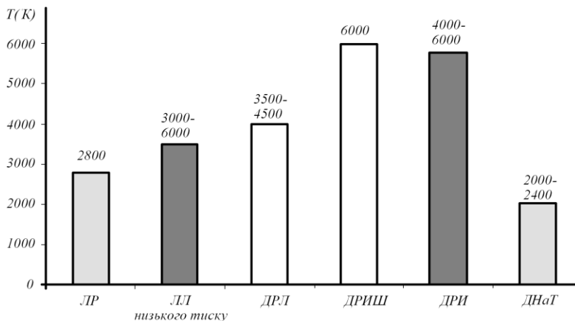
Рисунок 69 - Кольорова температура, T K
