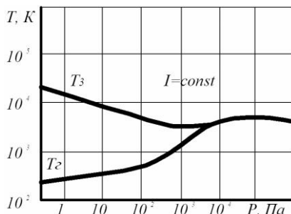
Рисунок 35 - Вимірювання температури газу T_g і електронної температури T_e при зміні тиску
