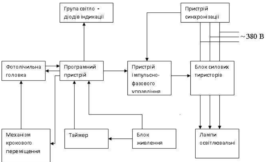
Рисунок 88 - Схема електрична структурна регулятора освітленості РОП-15-16-24
