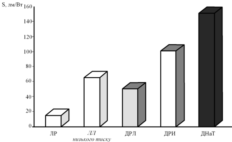
Рисунок 71 – Світлова віддача освітлювальних ламп, S , лм/Вт
