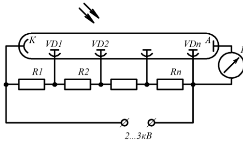
Рисунок 17 – Принципова схема вмикання фотоумножувача: К – катод; VD1...VD n – діоди; А – анод; R1... R n – резистори дільника; Г - вимірювальний прилад, гальванометр
