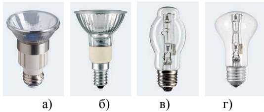
Рисунок 28 - Галогенні лампи: а) лампа MASTER PAR20E з відбивачем; б) лампа PAR16 Halogen A з відбивачем; в) лампа Halogen A Pro без відбивача; г) лампа Кrypton без відбивача
