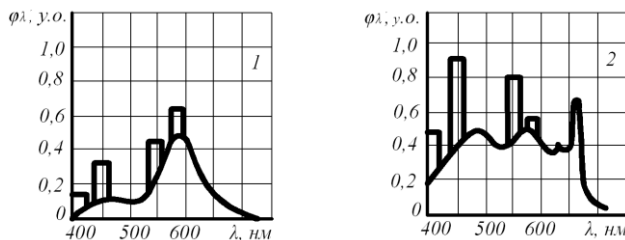
Рисунок 41 – Спектри випромінювання ламп: 1 – ЛБ; 2 – ЛДЦ
