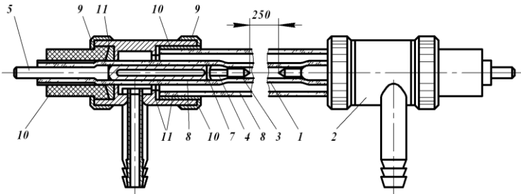
Рисунок 66 – Трубчаста ксенонова лампа:
