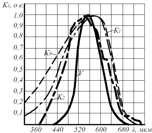
Рисунок 22 – Спектри чутливості селенових фотоелементів: К1 – фотоелемента люксметра Ю-117; К2 – теж з насадками КС; К3 – не корегованого фотоелемента; V – крива світності
