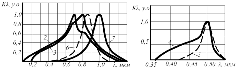
Рисунок 12 – Спектри чутливості фоторезисторів
