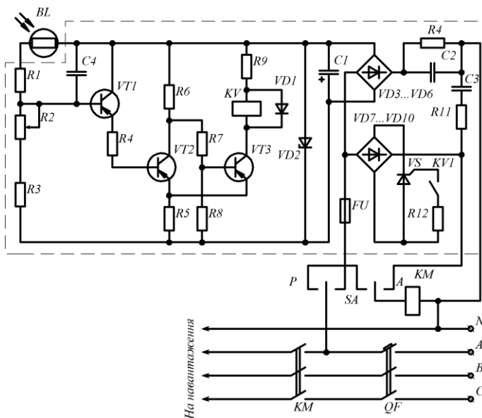
Рисунок 91 – Схема електрична принципова фотовимикача ФВ-2
