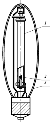
Рисунок 61 – Будова лампи ДНаТ: 1 – внутрішня керамічна розрядна трубка; 2 – вольфрамовий електрод; 3 – зовнішня колба
