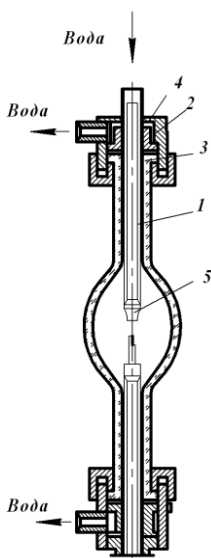
Рисунок 65 – Ксенонова лампа типу ДКСР
