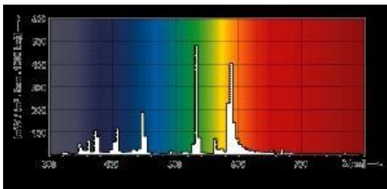
Рисунок 59 - Спектр випромінювання лампи ДРИ 400 HP1-T Plus
