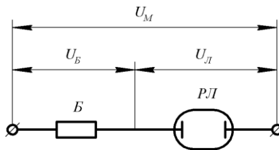
Рисунок 37 – Принцип включення РЛ в мережу: Б – баласт
