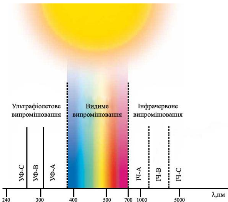
Рисунок 1 – Спектр електромагнітного випромінювання
