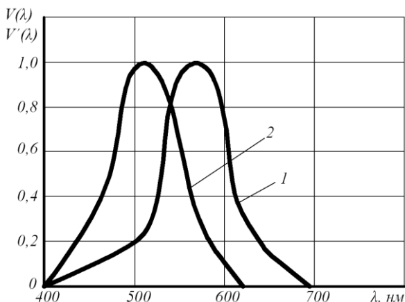
Рисунок 2 Середнє значення спектральної чутливості ока 1 - усереднена крива спектральної чутливості ока; 2 - крива спектральної чутливості ока в умовах нічного зору
