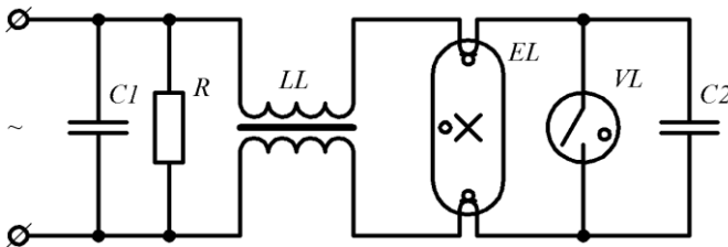
Рисунок 43 – Стартерна схема включення люмінесцентної лампи
