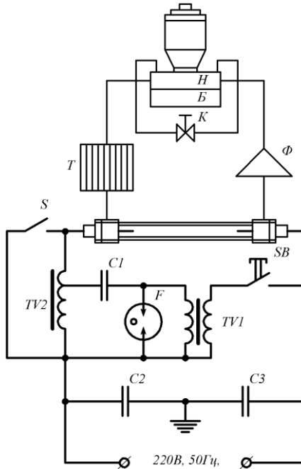
Рисунок 67 – Принципова спрощена схема пускового пристрою і система охолодження лампи ДКСТВ 6000
