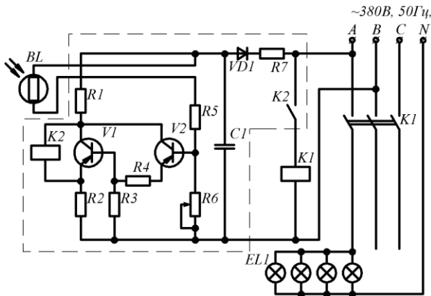
Рисунок 90 - Схема електрична принципова управління вуличним освітленням за допомогою фотореле ФР-2
