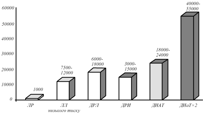
Рисунок 72 – Термін служби, t (год)
