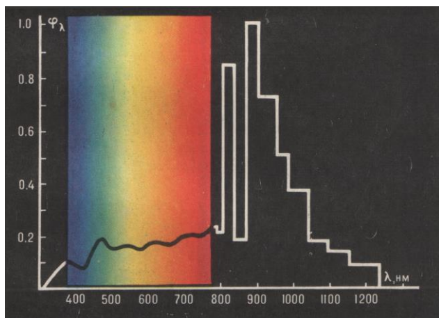
Рисунок 68 - Спектральна щільність випромінювання лампи ДКСТВ
