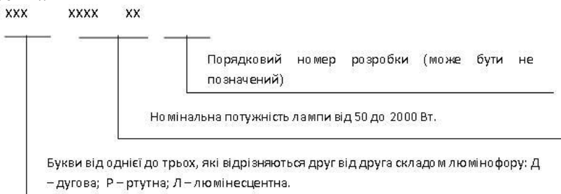
Рисунок 55 – Позначення люмінесцентних ламп високого тиску
