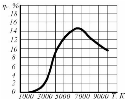
Рисунок 25 – Залежність світлового ККД від температури абсолютно чорного тіла
