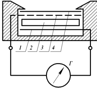
Рисунок 15 – Вентильний фотоелемент
