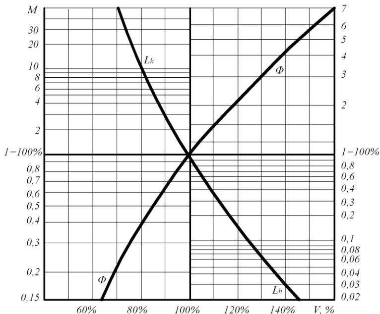
Рисунок 32 - Графік світлової віддачі та терміну служби в залежності від напруги галогенної лампи низької напруги
