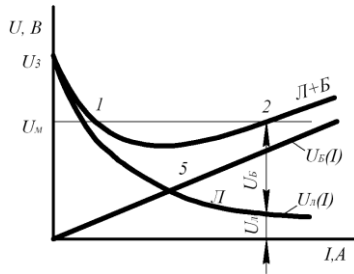
Рисунок 38 – ВАХ баласту РЛ і схеми лампи з баластом
