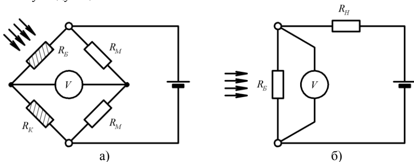
Рисунок 19 – Схеми включення болометрів: а) мостова; б) схема з навантажувальним опором
