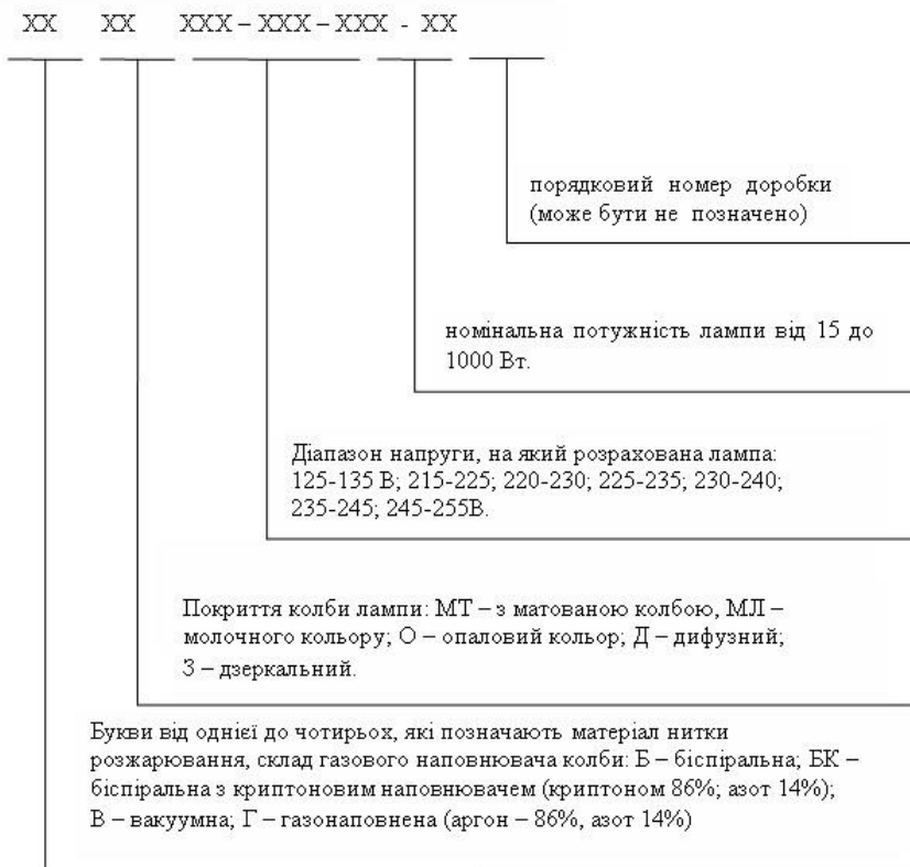
Рисунок 28 – Позначення лампи розжарювання загального призначення
