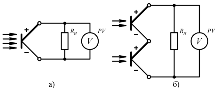
Рисунок 20 – Схема включення термоелектричних приймачів: а) термопара; б) термоелемент
