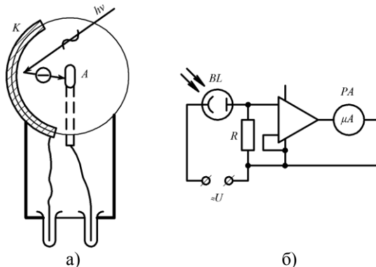
Рисунок 16 – Фотоелемент із зовнішнім фотоелементом: а) конструкція; б) принципова електрична схема
