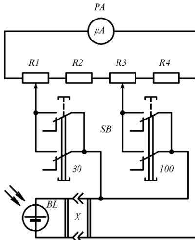
Рисунок 23 – Принципова електрична схема люксметра Ю-116
