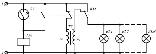
Рисунок 86 – Схема пристрою для обмеження пускових струмів ЛР
