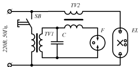
Рисунок 58 – Схема включення лампи ДРИ
