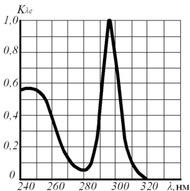
Рисунок 4 - Спектр еритемної дії ультрафіолетового випромінювання
