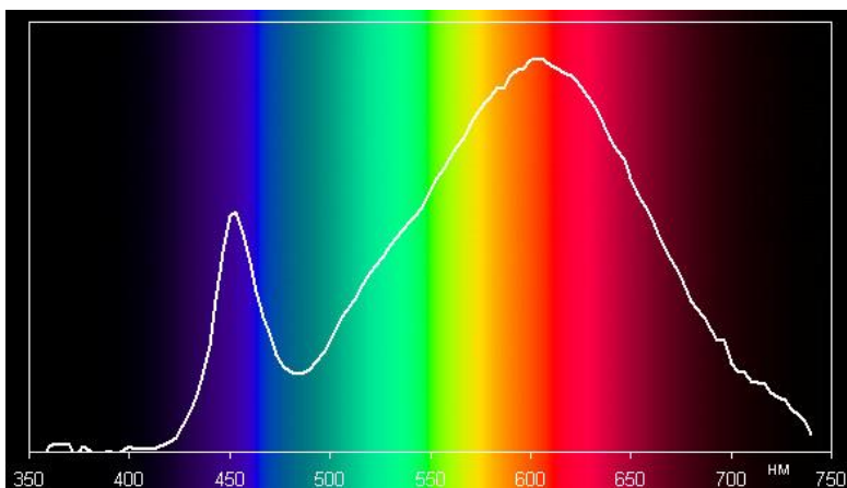
Рисунок 75 – Спектр випромінювання світлодіодної лампи Thomson RTBL-RE60-CW (T11CW)
