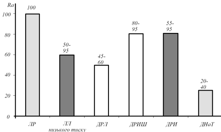
Рисунок 70 – Індекс кольоропередачі (Ra)
