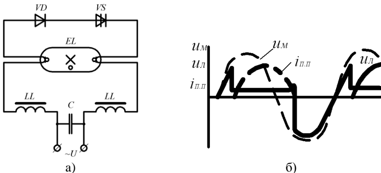
Рисунок 49 – а) Схема включення ЛЛ з напівпровідниковим стартером; б) Осцилограми миттєвих значень напруги і струму при запалюванні люмінесцентної лампи за допомогою динистора. VS - динистор; VD – діод; LL – дросель; EL – люмінесцентна лампа
