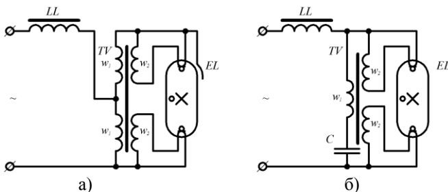
Рисунок 50 – а) Безстартерна схема включення ЛЛ з розжарювальним трансформатором гарячого запалювання: EL – люмінесцентна лампа; LL – дросель; TV - розжарювальний трансформатор; б) Резонансна безстартерна схема включення ЛЛ з розжарювальним трансформатором холодного запалювання: С – конденсатор; w_1 – первинна обмотка трансформатора; w_2 – вторинна обмотка трансформатора
