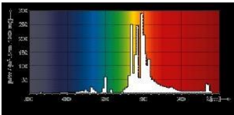
Рисунок 63 - Спектр випромінювання лампи ДНаТ 250 SON-T В
