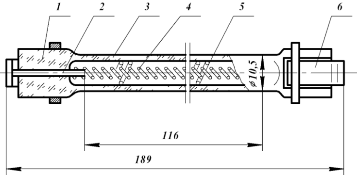
Рисунок 29 - Лампа кварцова галогенна КГ220-1000: 1 - плоскоштамповані ніжки лампи; 2 – молибденовий електрод; 3 – кварцова колба; 4 – моно спіраль тіла накали; 5 – вольфрамові тримачі; 6 – плоскі контактні поверхні
