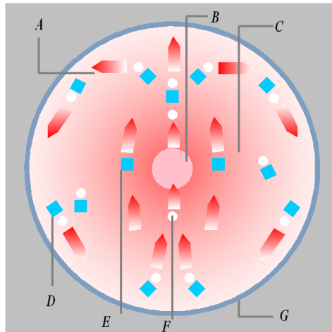
Рисунок 30 - Регенеративний йодний цикл: А) – температура нижче 1400 °С; В) – вольфрамова нитка розжарювання; С) – температура більше 1400 °С; D) – вольфрамовий галоген; Е) – галогени; F) – частинки вольфраму; G) – скляна колба
