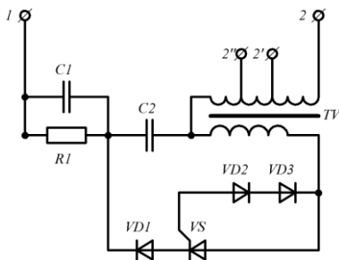
Рисунок 62 - Принципова електрична схема пристрою імпульсного запалюючого універсального типу УІЗУ
