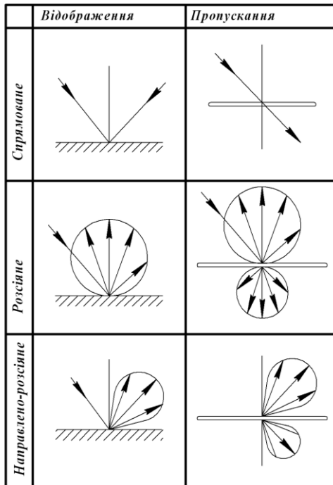
Рисунок 10 – Різновидності відбивання і пропускання потоку оптичного випромінювання
