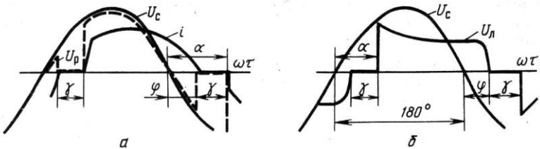
Рисунок 84 – Осцилограми, які отримані в колі з тиристорним регулюванням: а) напруги; б) струму
