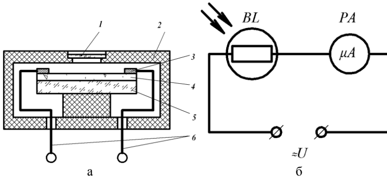
Рисунок 12 – Конструкція (а) і схема включення фото резистора (б): 1 - захисний прозорий шар; 2 - корпус; 3 – електрод; 4 - шар напівпровідника; 5 - підкладка (ізолятор); 6 - виводи
