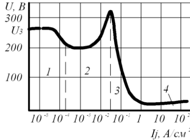
Рисунок 36 – ВАХ газового провідника:
