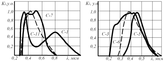
Рисунок 18 – Спектри чутливості фотоелементів із зовнішнім фотоелементом
