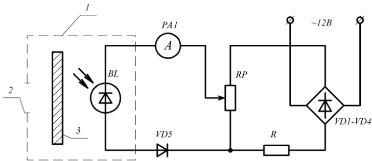
Рисунок 13 – Схема вимірювача опроміненості з фотодіодом:
