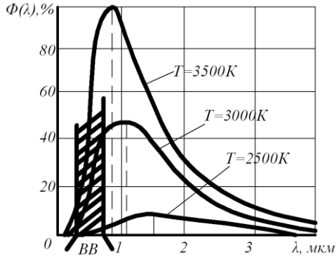
Рисунок 24 - Спектральна щільність випромінювання абсолютно чорного тіла при нагріванні його до різних температур
