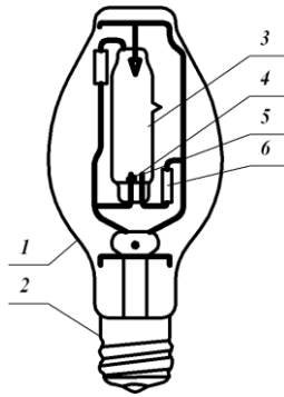
Рисунок 52 – Лампа високого тиску ДРЛ:
