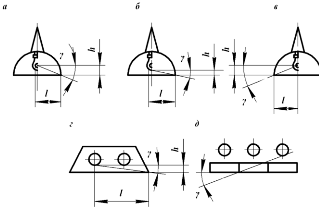
Рисунок 78 – Захисний кут світильника, який створюється відбивачами (а, б, в, г) і екранною решіткою (д):
