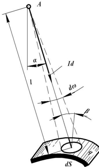
Рисунок 9 - До висновку відношення між силою світла і освітленістю
