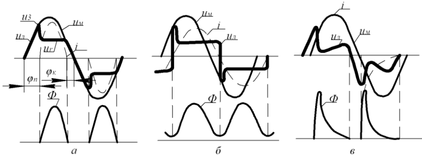
Рисунок 39 – Осцилограми миттєвих значень напруги, струму і світлового потоку газорозрядної лампи:
