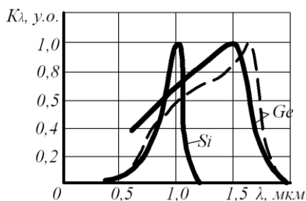
Рисунок 14 - Спектри чутливості фотодіодів на основі германія (Ge) і кремнія (Si)
