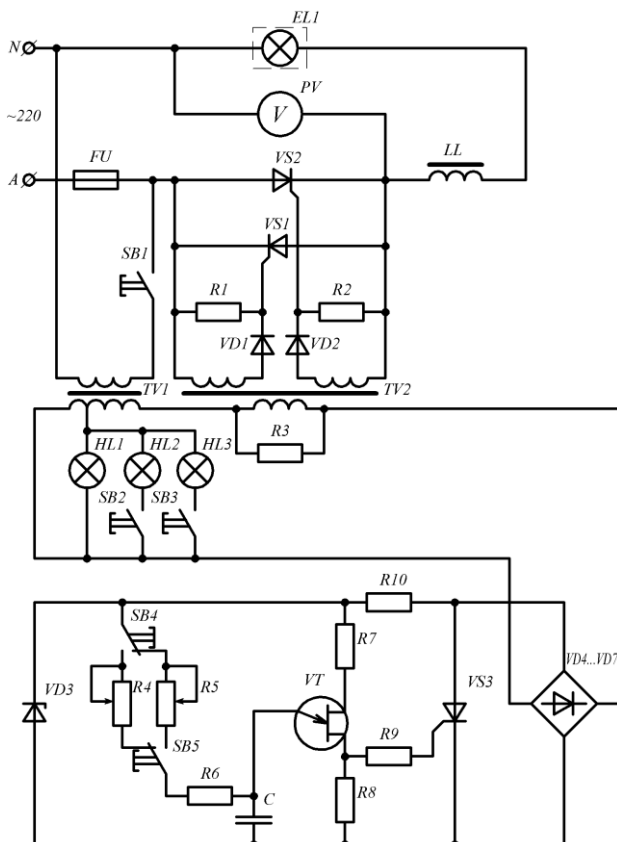
Рисунок 87 – Схема електрична принципова установки «ТІРОС»
