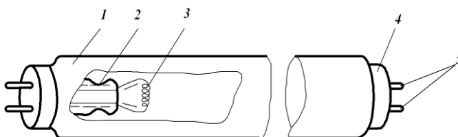
Рисунок 40 – Конструкція люмінесцентної лампи загального призначення в розрізі
