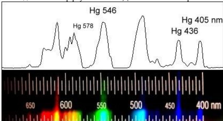
Рисунок 53 - Видимий спектр ртутної лампи ДРЛ
