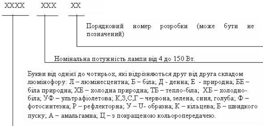
Рисунок 42 – Позначення люмінесцентних ламп низького тиску
