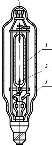
Рисунок 57 – Будова лампи ДРИ: 1 – внутрішня кварцова колба; 2 – електроди; 3 – зовнішня колба
