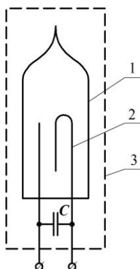
Рисунок 44 – Стартер:
