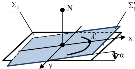
Рис. 1. Положення джерела аероіонного випромінювання і нахиленої площини
