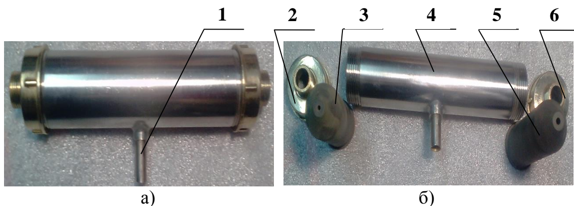
Рис. 1. Камера струминного гомогенізатора молока щілинного типу: а) у зборі, б) внутрішня будова: 1 – патрубок подачі продукту з ємності з вершками; 2 – патрубок подачі знежиреного молока; 3 – конфузор; 4 – корпус камери струминного диспергатора молока щілинного типу; 5 – дифузор; 6 – патрубок для відведення гомогенізованого та нормалізованого за жирністю молока
